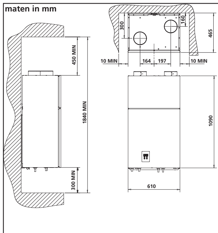
Fig.5 Maatschets Ecolution® Combi 50
