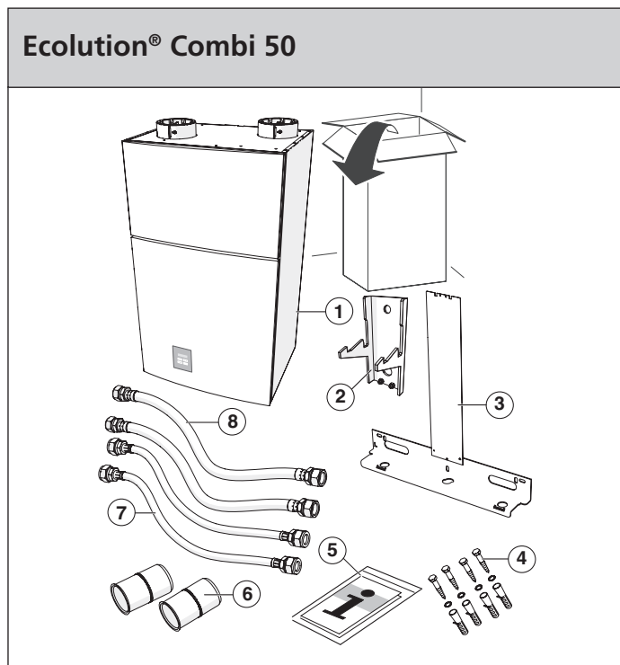
Fig. 1 Leveringsomvang Combi 50
