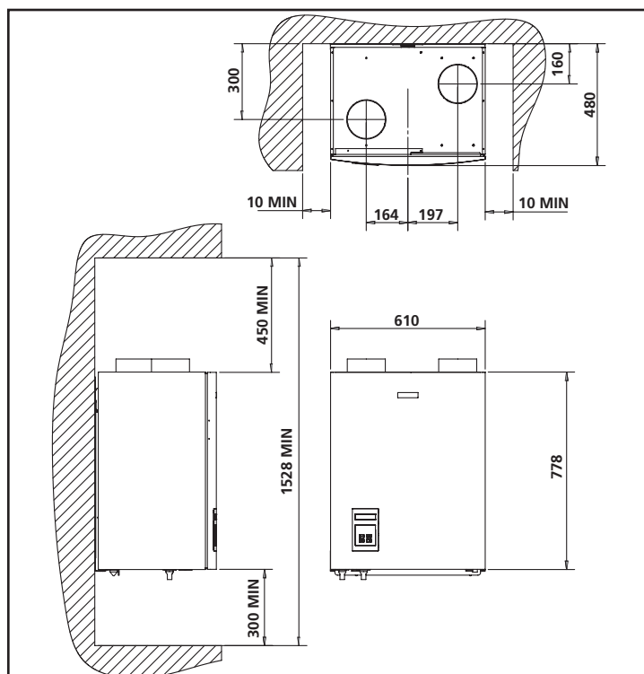
Fig.6 Maatschets Ecolution® Solo
