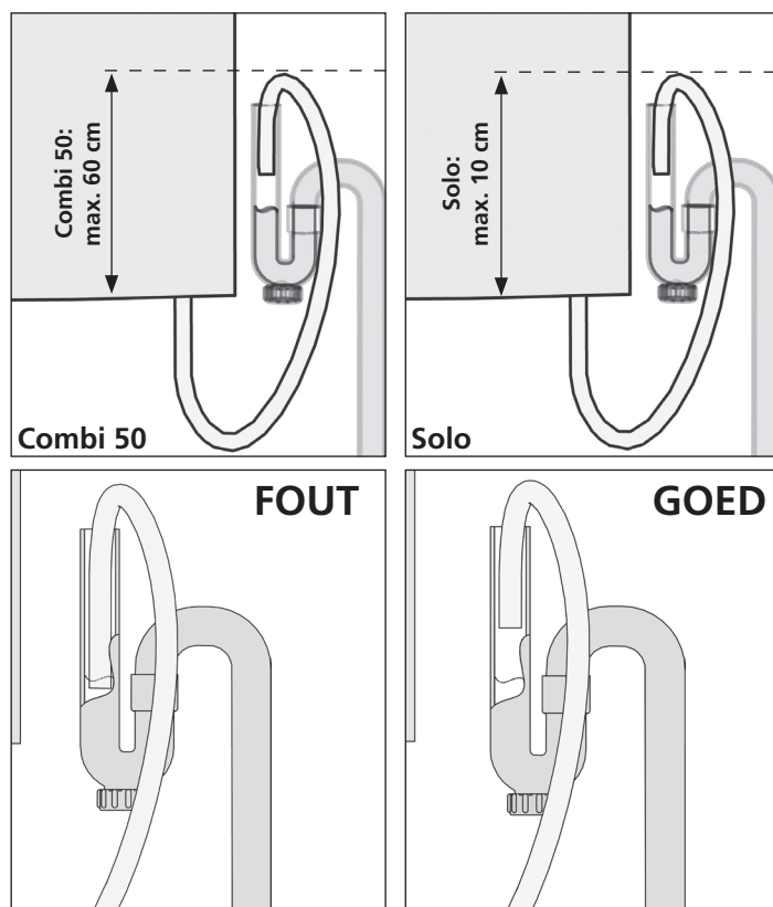
Fig. 10 Condensafvoer
