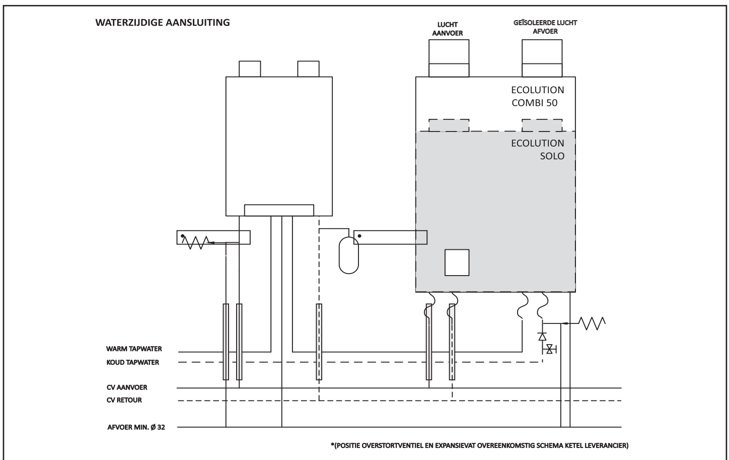
Fig. 7 Basisschema
