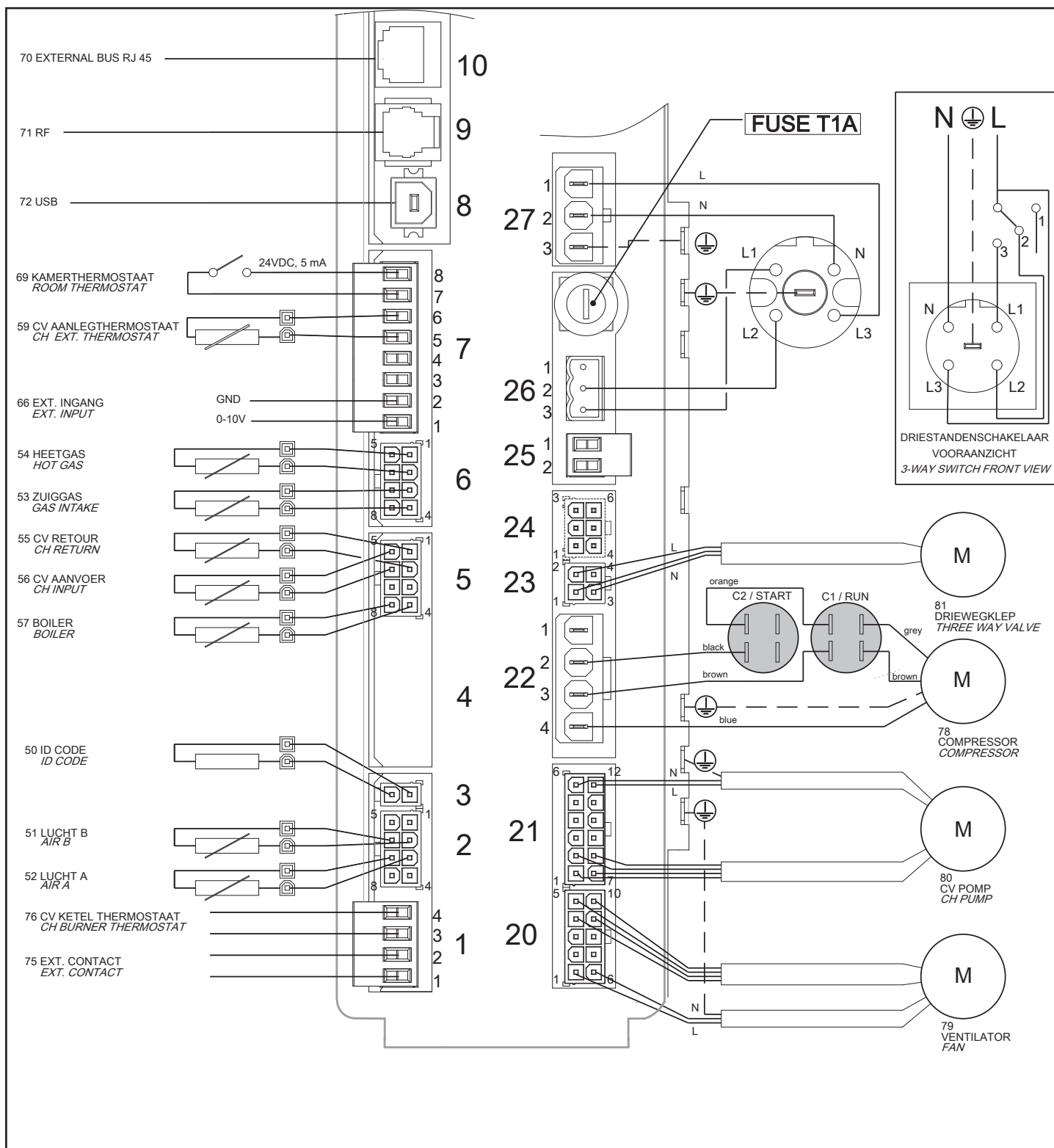
Fig. 11 Elektrisch schema
